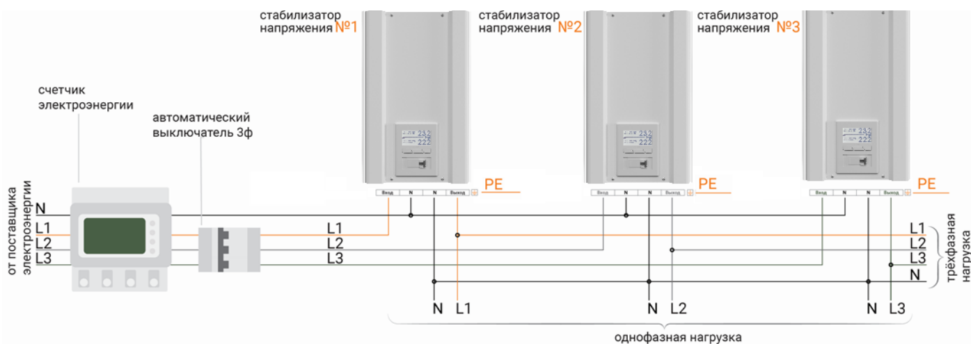
Рисунок 4. Схема подключения стабилизатора к трёхфазной сети
