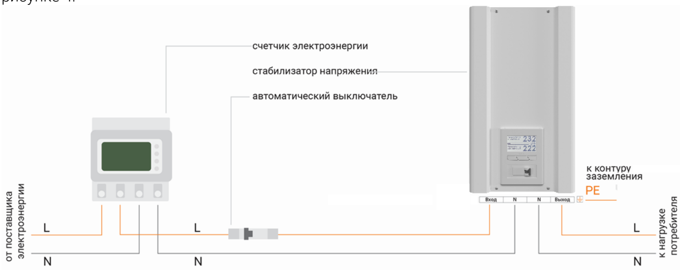
Рисунок 3. Схема подключения стабилизатора к однофазной сети
